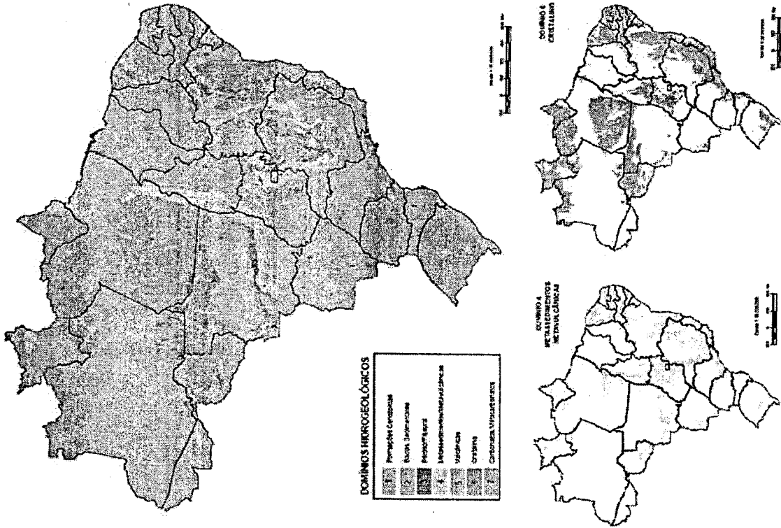
Figura 8 – Domínios Hidrogeológicos do Brasil - Todos os domínios; Domínio 4 (Metassedimentos/Metavulcânicas); e Domínio 6 (Cristalino).
